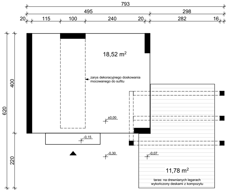
RZUT PARTERU
