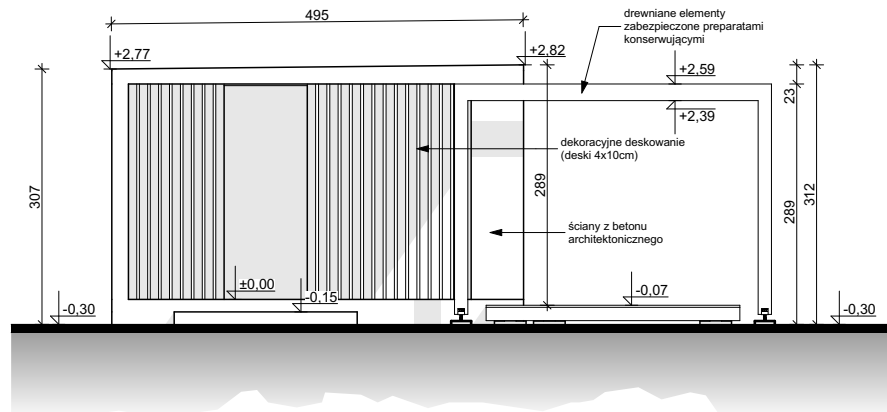
ELEWACJA FRONTOWA
