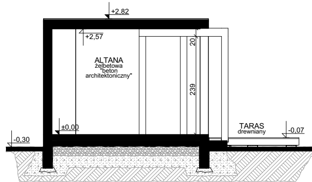
PRZEKRÓJ A-A
